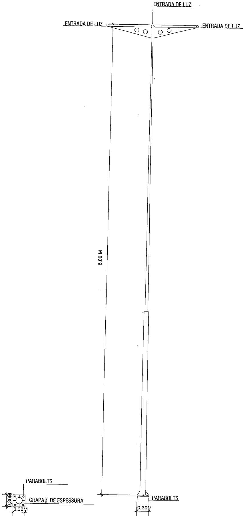
VISTA DE FRENTE COM COTAS
