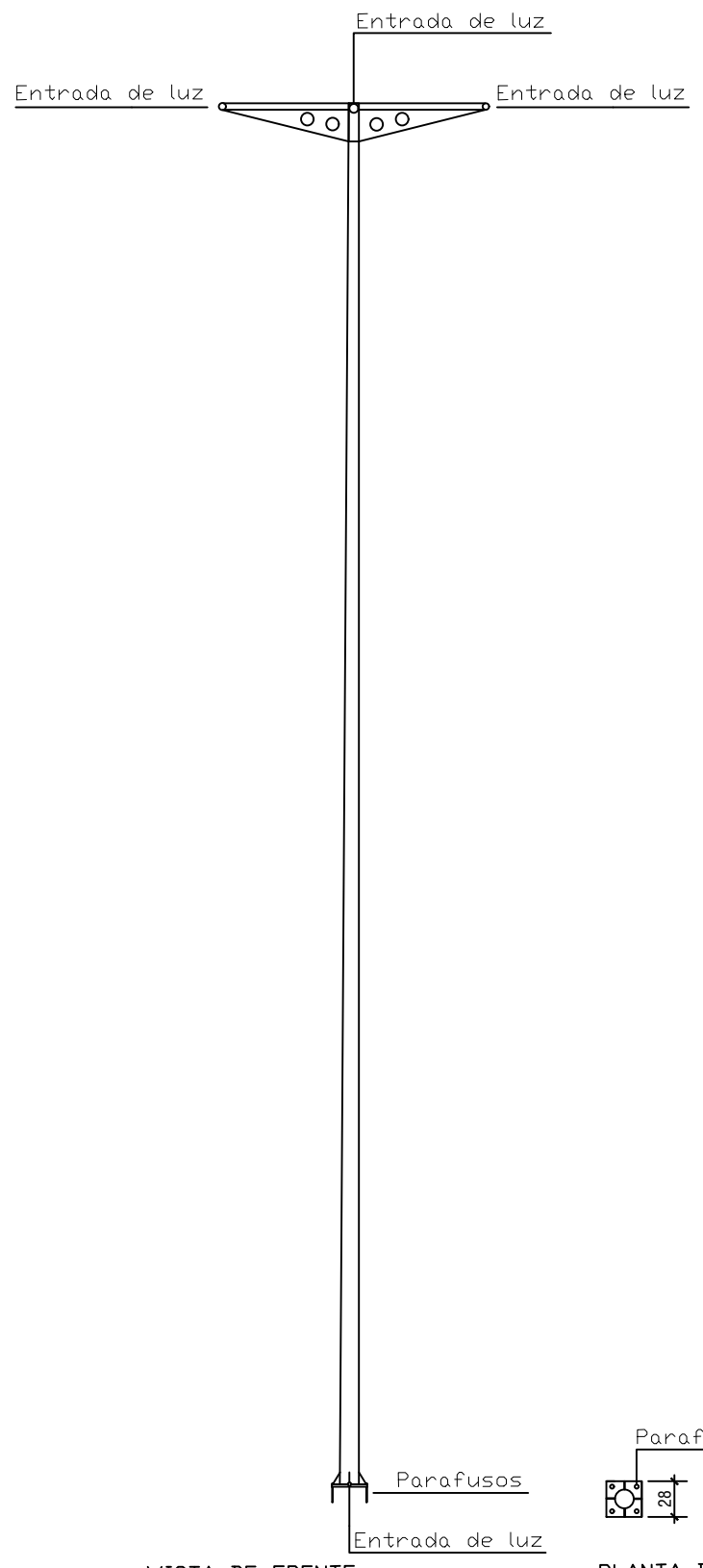
VISTA DE FRENTE
