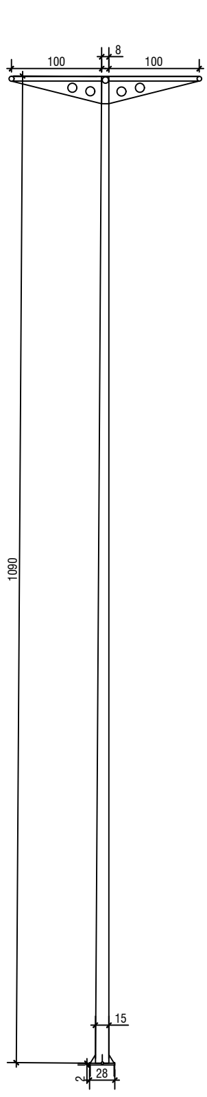
VISTA DE FRENTE COM COTAS
