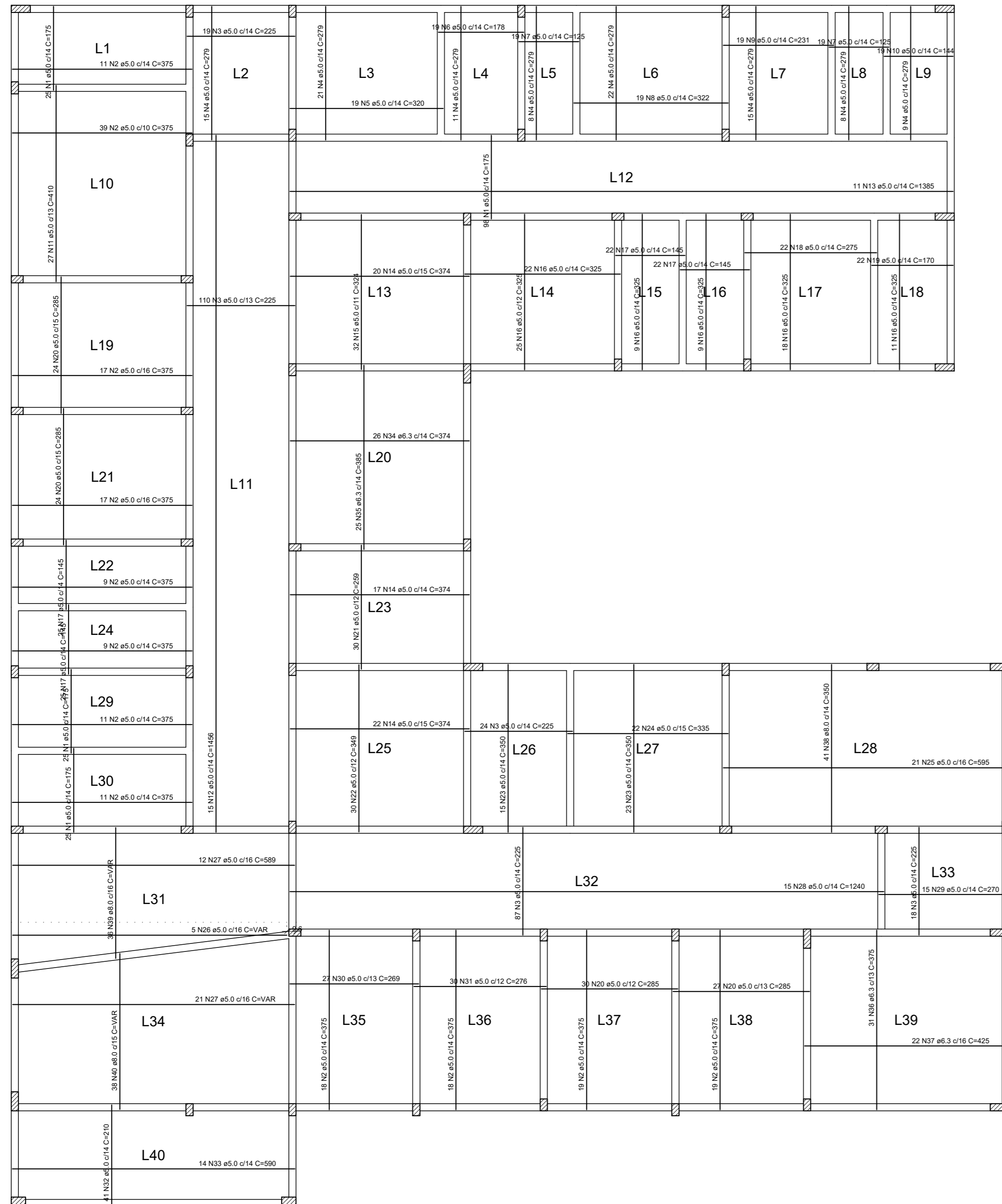
Armação positiva das lajes do pavimento Térreo escala 1:50
