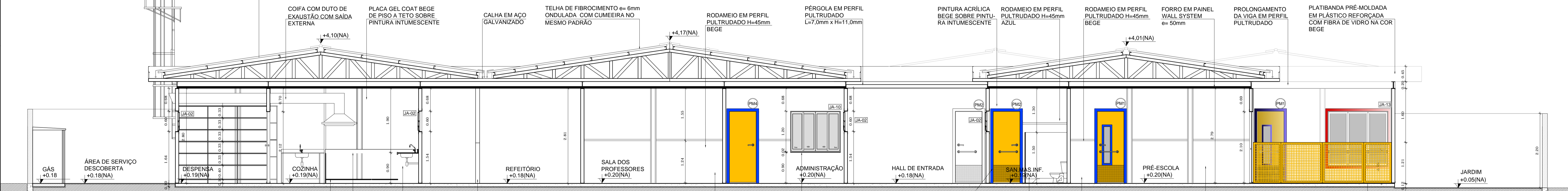
2 CORTE AA ESCALA 1:50
