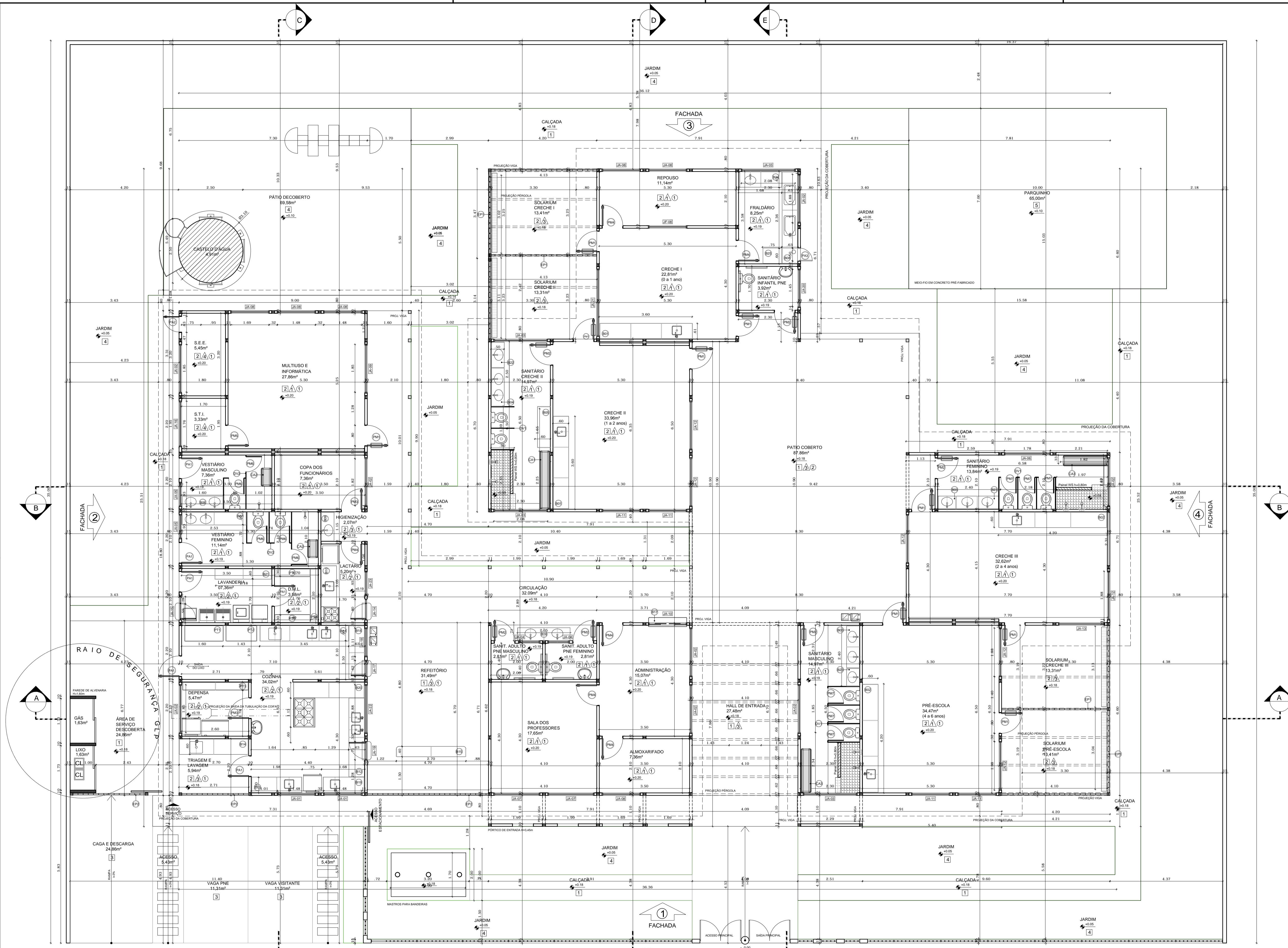
1 PLANTA BAIXA ESCALA 1:75
