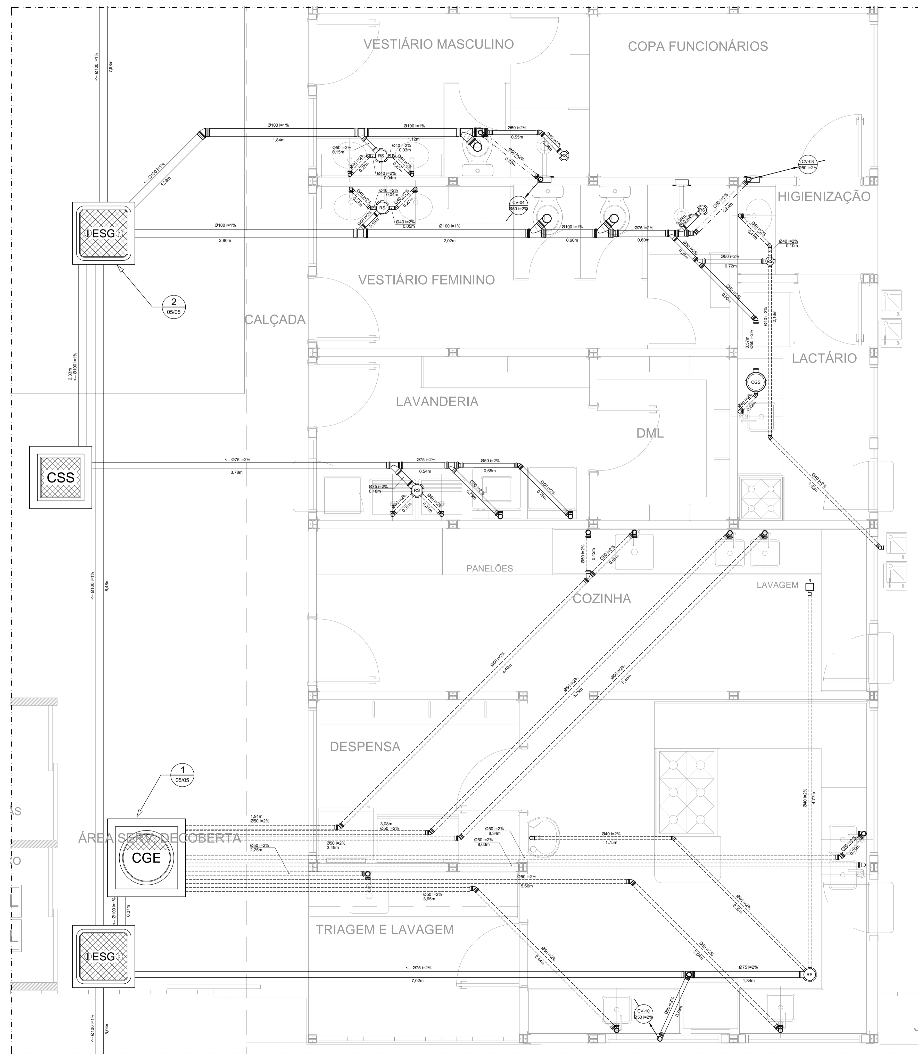
1 AMPLIAÇÃO 01 ESC.: 1/20
