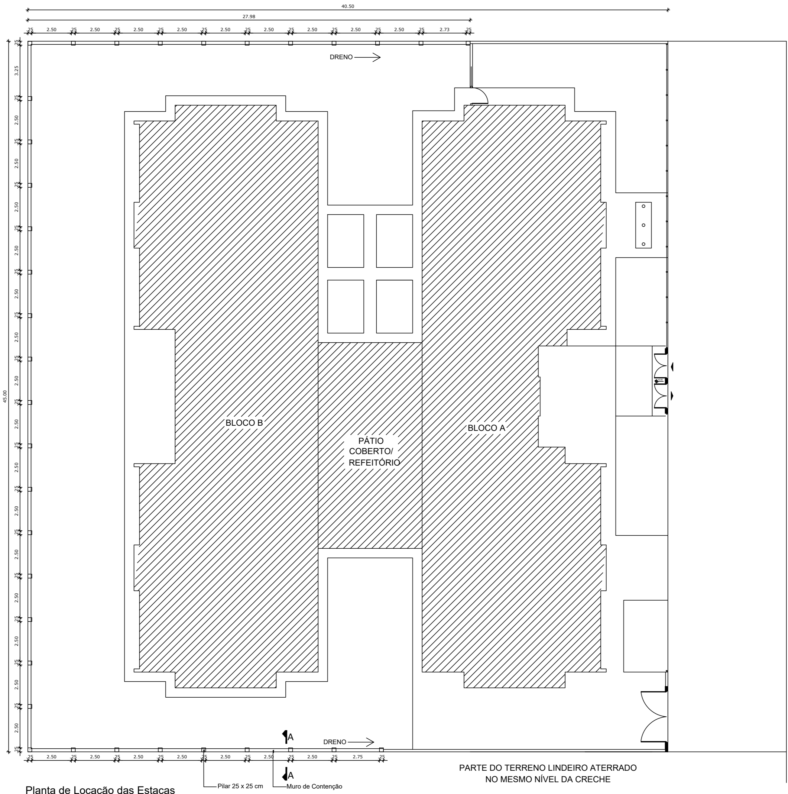
Planta de Localização das Estacas ESCALA 1/75
