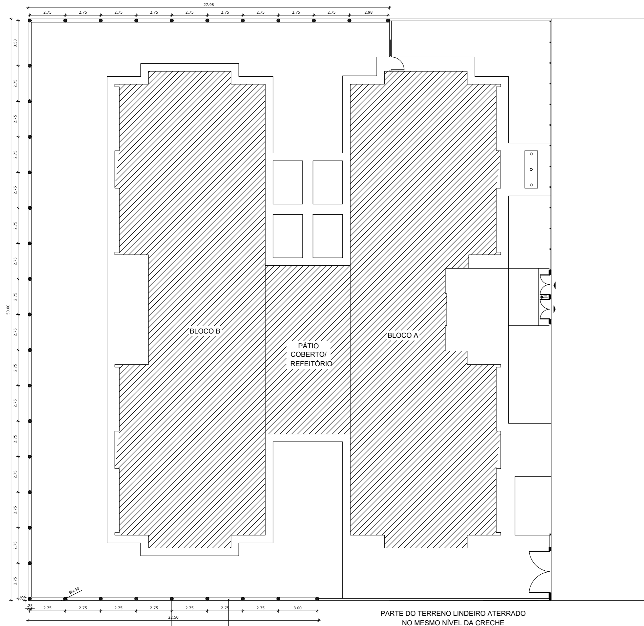
Planta de Locação das Estacas ESCALA 1/75
