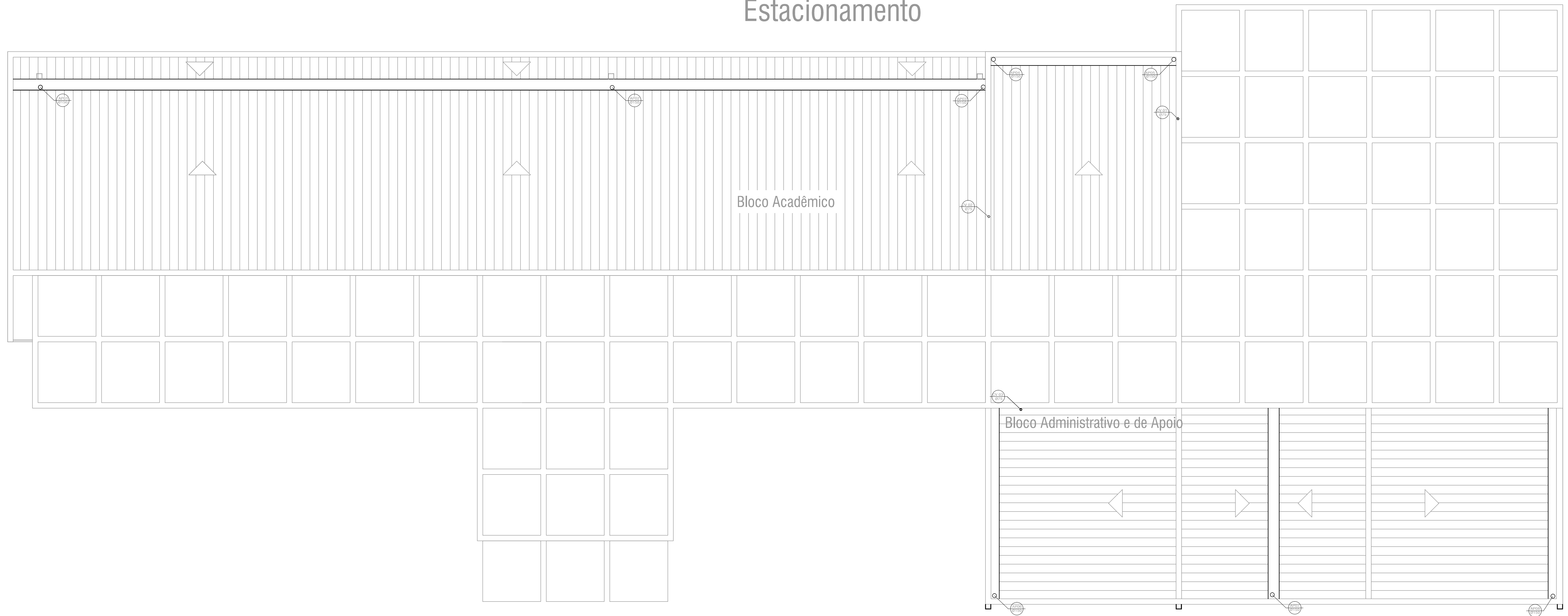
Projeto Hidrossanitário - Cobertura Esc.: 1/50
