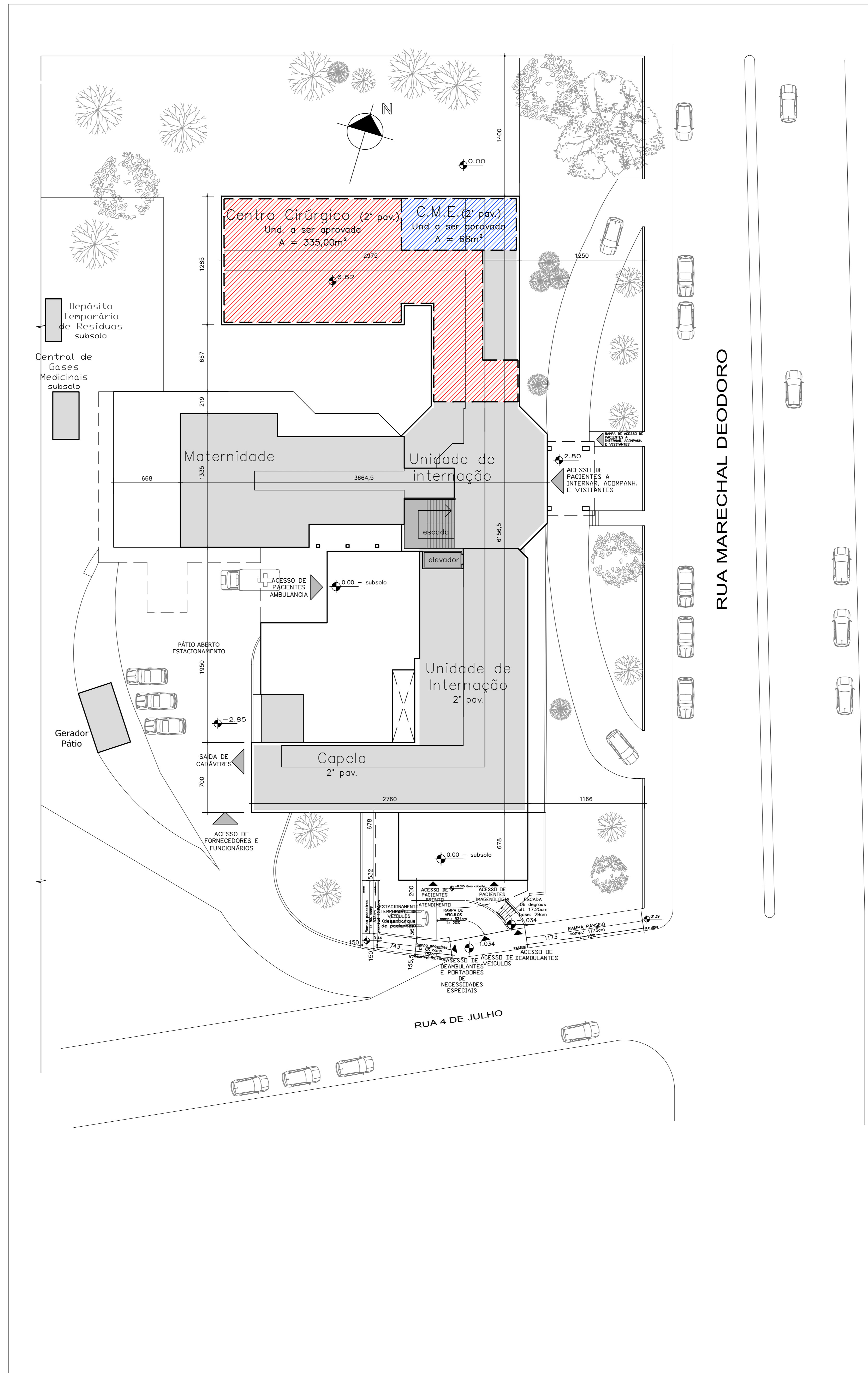
IMPLANTAÇÃO ESC.: 1/200
