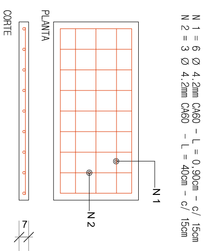
DETALHE FERRAGEM – TAMPA SEM ESCALA
