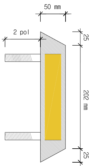
VISTA LATERAL SEM ESCALA
