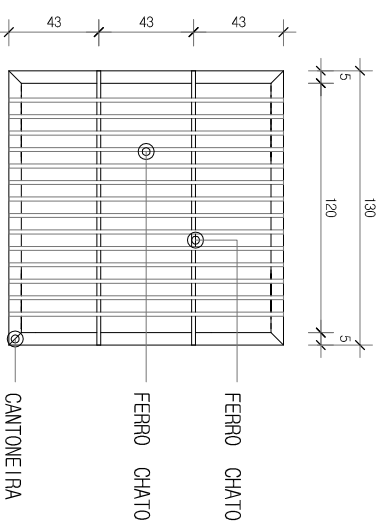
Planta Baixa – Caixa Gradeada (1,20 x 1,20) SEM ESCALA
