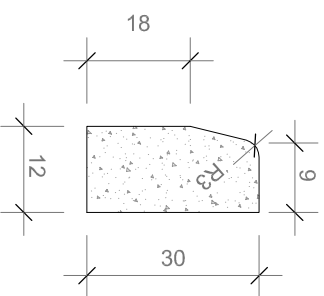
VISTA LATERAL SEM ESCALA
