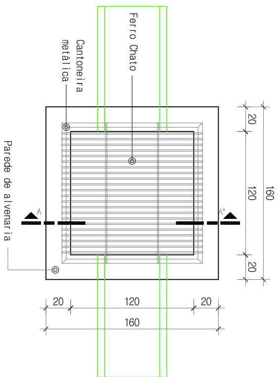
Planta Baixa – Caixa Gradeada (1,20 x 1,20) SEM ESCALA
