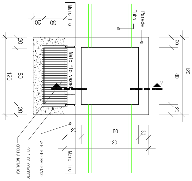
PLANTA BAIXA – CAIXA COLETORA COMBINADA 0,80X0,80 int. SEM ESCALA
