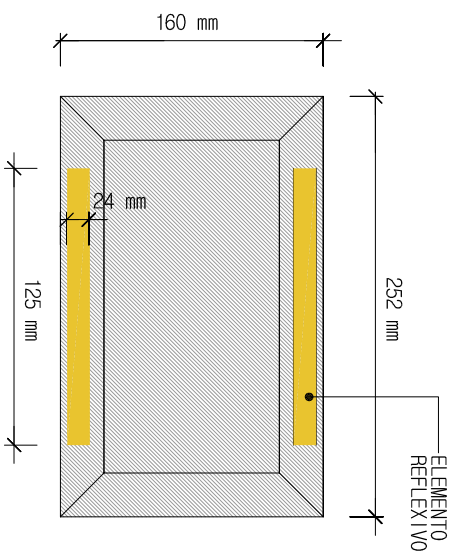
VISTA SUPERIOR SEM ESCALA
