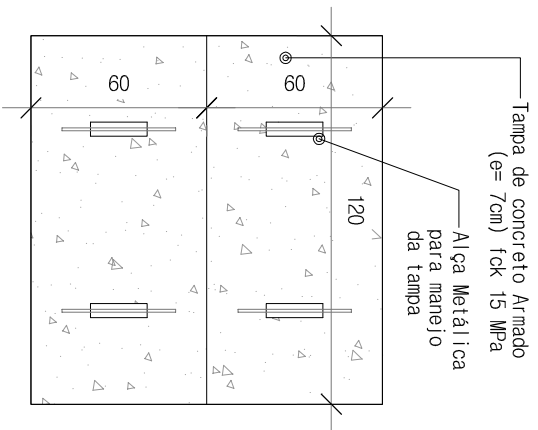
PLANTA BAIXA – TAMPA SEM ESCALA
