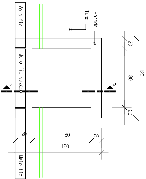
PLANTA BAIXA – CAIXA BLS : 0,80x0,80 int. SEM ESCALA
