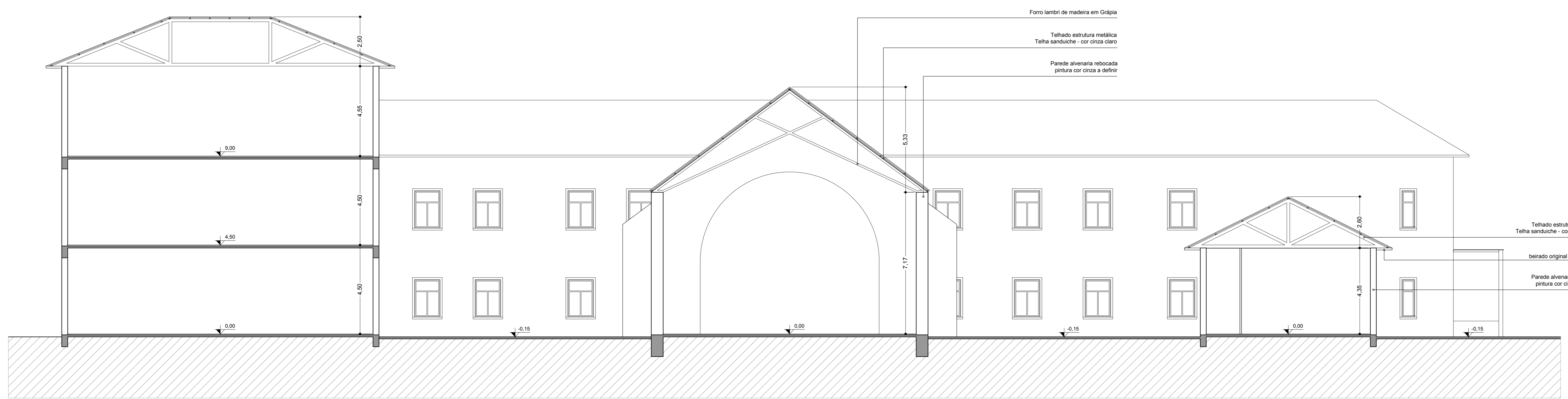
CORTE CC
